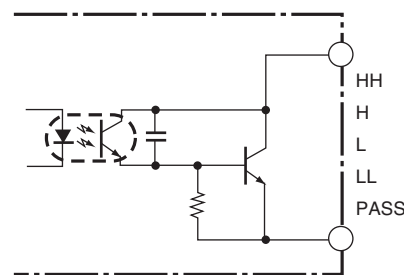
晶体管输出时 (NPN集电极开路)
