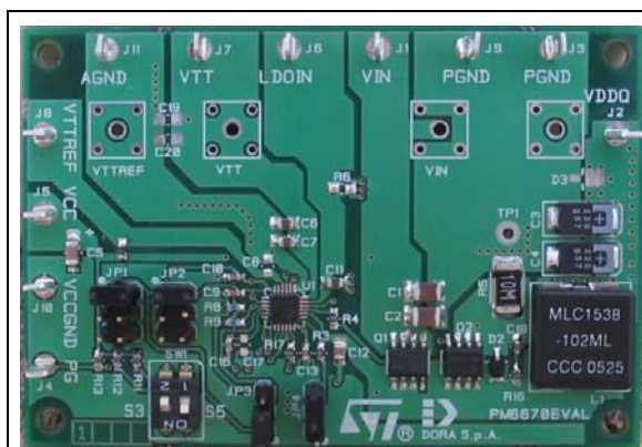
STEVAL-ISA051V2
