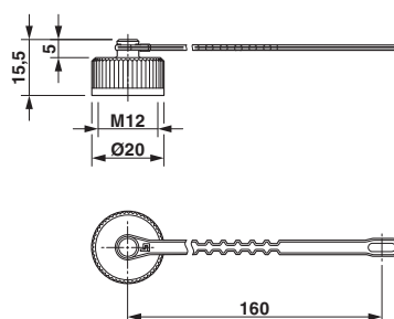
尺寸图
