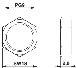
尺寸图
