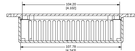
SECTION D-D
