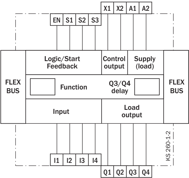
接线图
