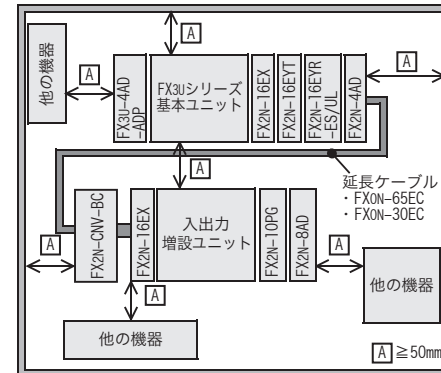
増設延長ケーブルを使用し2段に配置した構成
