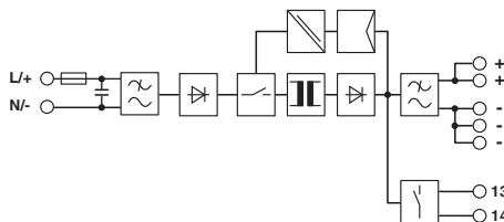
结构框图
