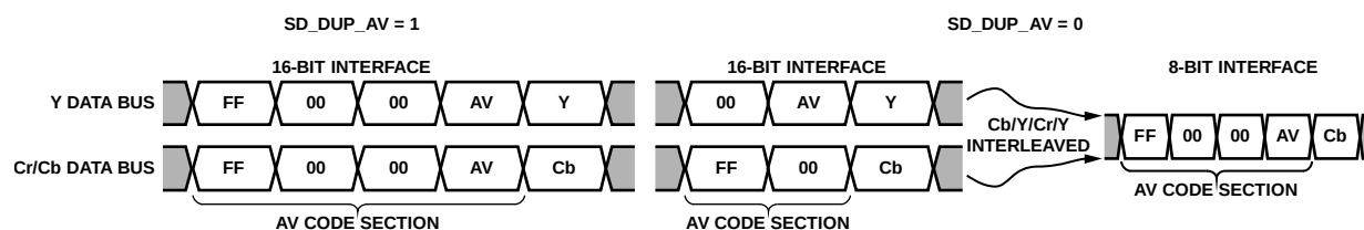
Figure 32. AV Code Duplication Control (64-Lead LQFP Only)
