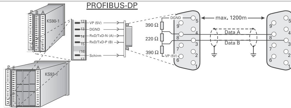
Fig.:2 PROFIBUS-DP connection
