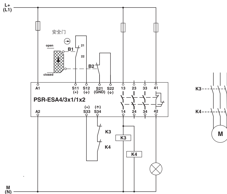
电路图
