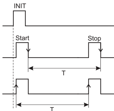
Bild 2-1: Zeit-/Wegmessprinzip
