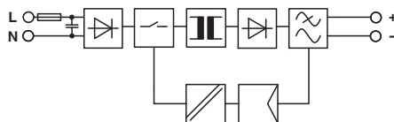
结构框图
