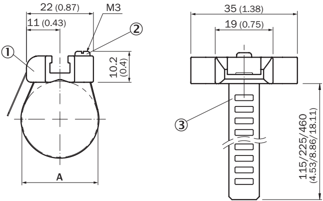
尺寸图 (尺寸单位: mm)
