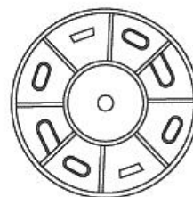
Takfäste
