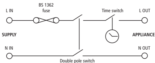
Fig. 3 Internal Schematic of FST17A / FST11A
