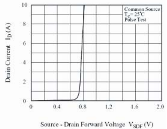
Fig6. I_S - V_{SDF}
