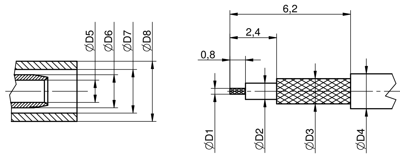
Kabelzuschnitt Stripping dimension
