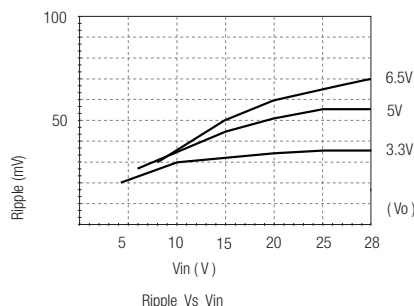
R-74xx Ripple VS Vin
