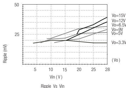
R-72xx / R-73xx Ripple VS Vin
