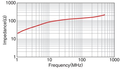
HF70RU10X20X5S
