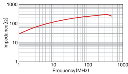
HF70RU26X29X13S
