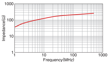
HF70RH13X20X5
