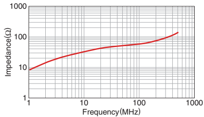
HF70RH14X14X10
