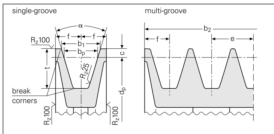
Groove section
