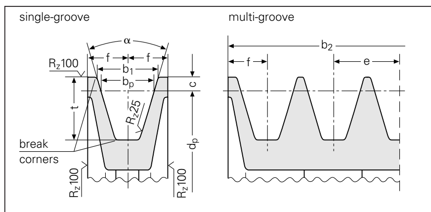
Groove section
