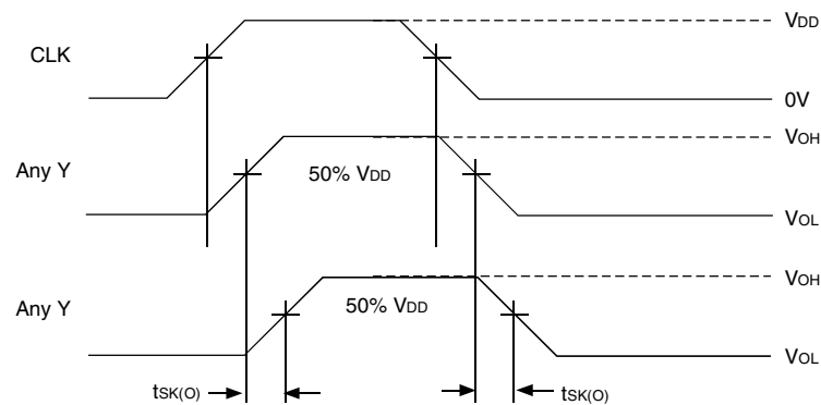
Output Skew
