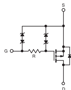
P-Channel MOSFET
