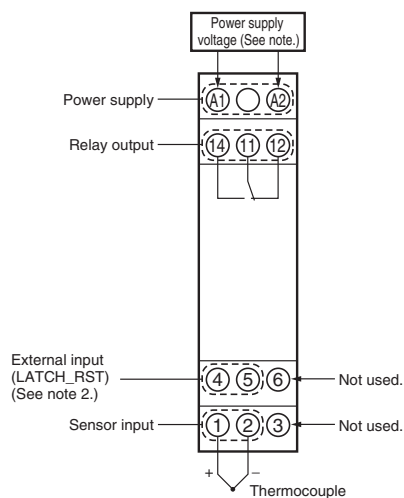
K8AB-TH12S
