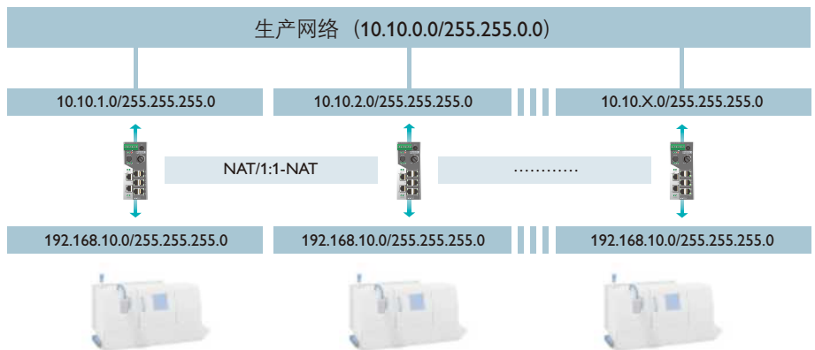
采用具有NAT功能的交换机进行自动IP地址转换
