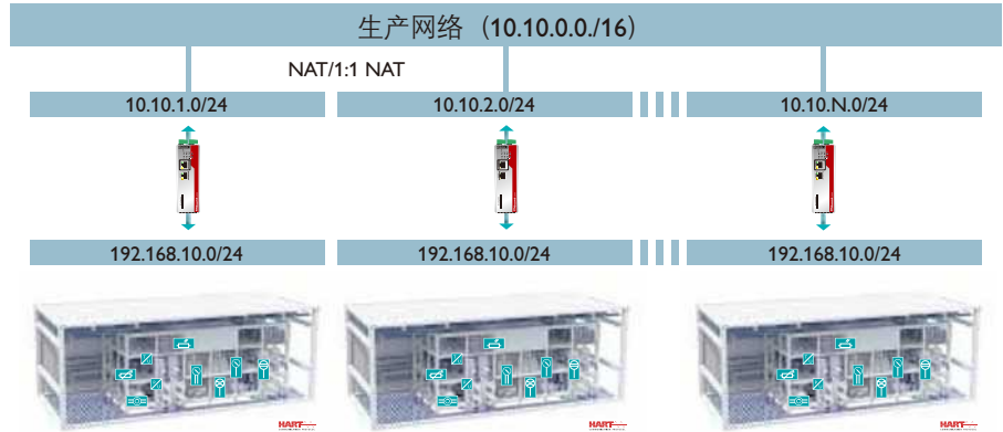
通过1:1 NAT功能，可以访问具有相同IP地址的系统部件
