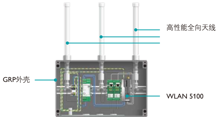
防爆区的WLAN解决方案
