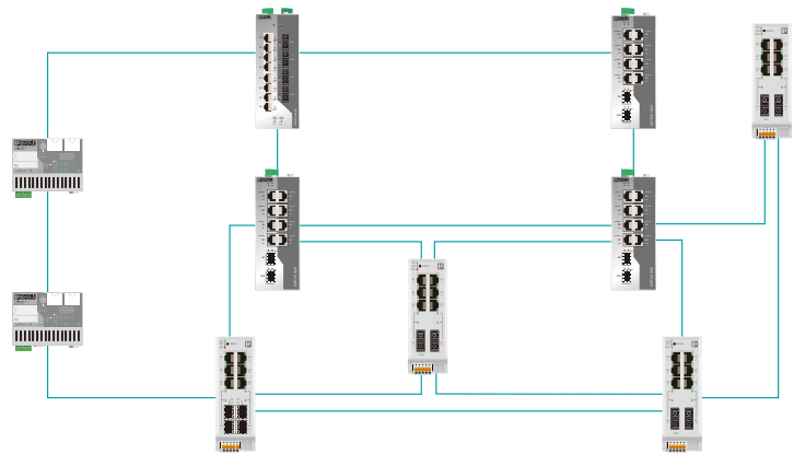
用于高网络可用性的RSTP冗余
