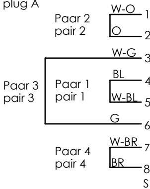
Stecker A plug A
