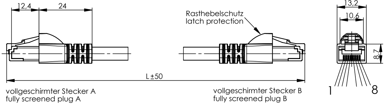
Stecker B plug B
