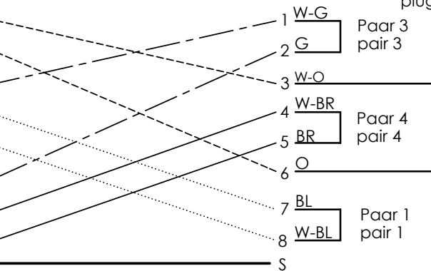
Stecker B plug B
