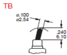
ESD PLASTIC ACTUATOR
