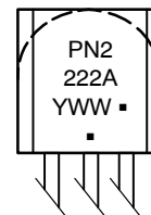
PN2222A
