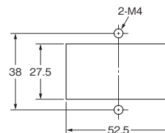
取り付け穴加工寸法
