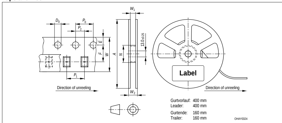
W P_0 P_1 P_2 D_0 E F 8^{+0.3}_{-0.1} 4 \pm 0.1 ( 0.157 \pm 0.004 ) 2 \pm 0.05 ( 0.079 \pm 0.002 ) 2 \pm 0.05 ( 0.079 \pm 0.002 ) 1.5 \pm 0.1 ( 0.059 + 0.004 ) 1.75 \pm 0.1 ( 0.069 \pm 0.004 ) 3.5 \pm 0.05 ( 0.138 \pm 0.002 )
