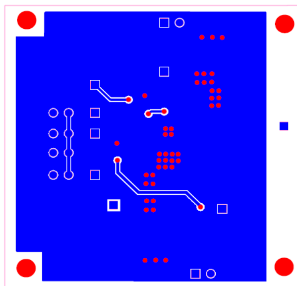
Figure 19. Bottom Layer
