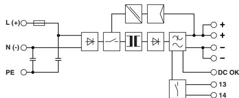
结构框图
