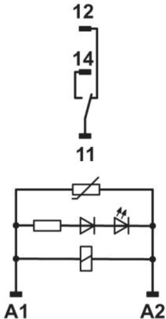
电路图
