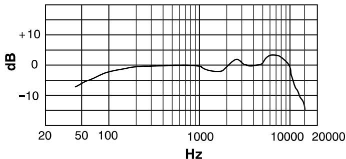
TIPICA RISPOSTA IN FREQUENZA
