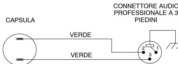
CONNESSIONI INTERNE
