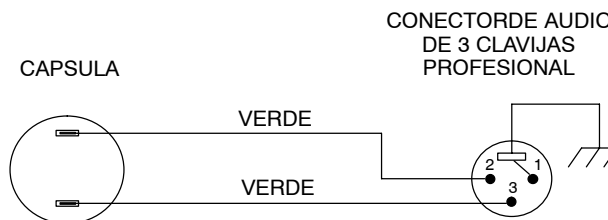
CONEXIONES INTERNAS
