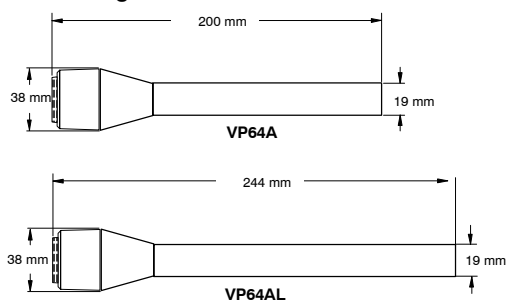
DIMENSIONES GENERALES FIGURA 3
