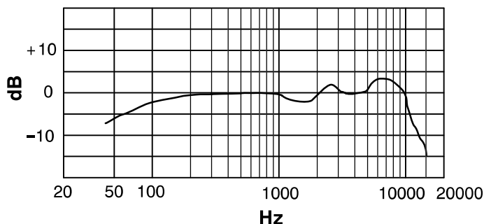
RESPUESTA DE FRECUENCIA TÍPICA
