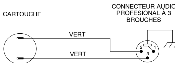
BRANCHEMENTS INTERNES
