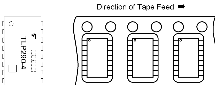
Fig. 15.3.1.1 Device Orientation
