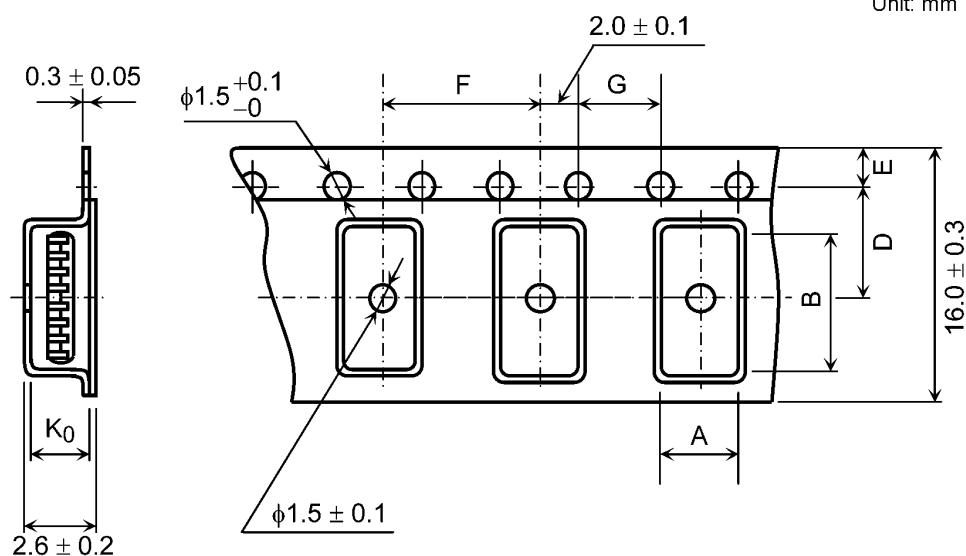
Fig. 15.3.5.1 Tape Dimensions
