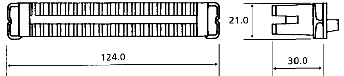
10 Pair Module
