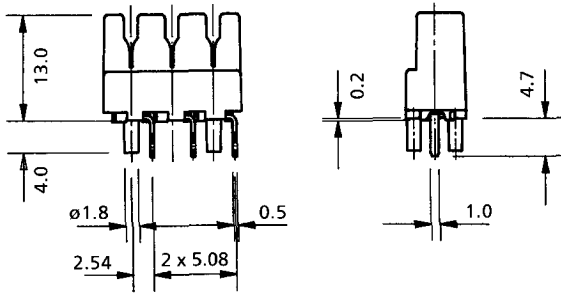
3 Way PCB Connection Module
