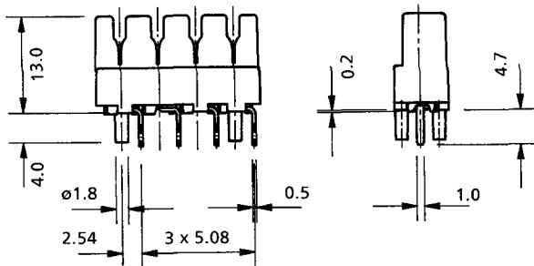
4 Way PCB Connection Module
