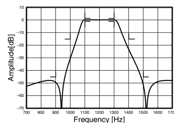
CF-4FPA 1200Hz
