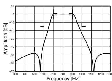
CF-4FPA 800Hz
