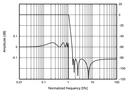
Amplitude
