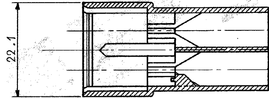
SEZ. A-A
