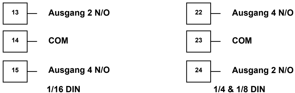
Bild 26 - Options-Steckplatz 2 - Doppelrelais-Modul
