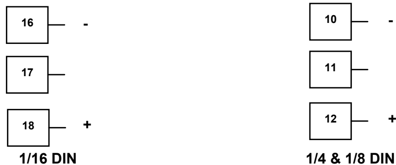
Bild 33 - Options-Steckplatz 3 - Messumformer-Stromversorgungsmodul
