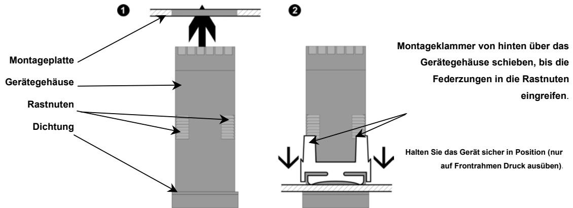
Bild 3 - Geräte-Einbau
