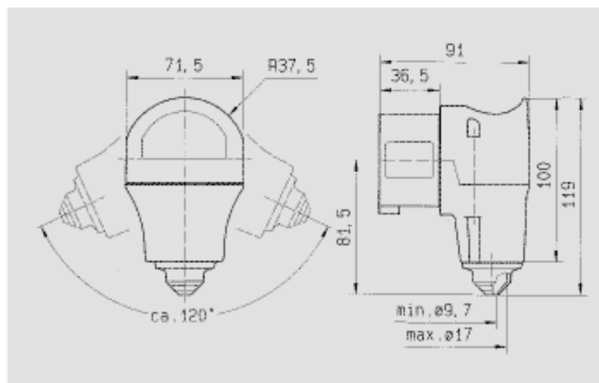
Zeichnung 2 MB 208 Maße in mm
