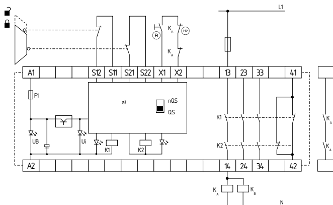
Fig. 4 a) Logic
