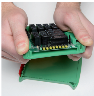
Estrazione della scheda elettronica. Removing the pcb.
