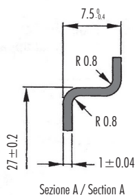
Sezione A / Section A
