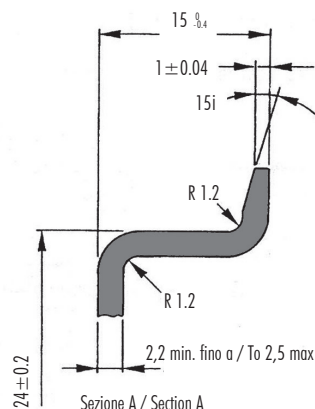
Sezione A / Section A
