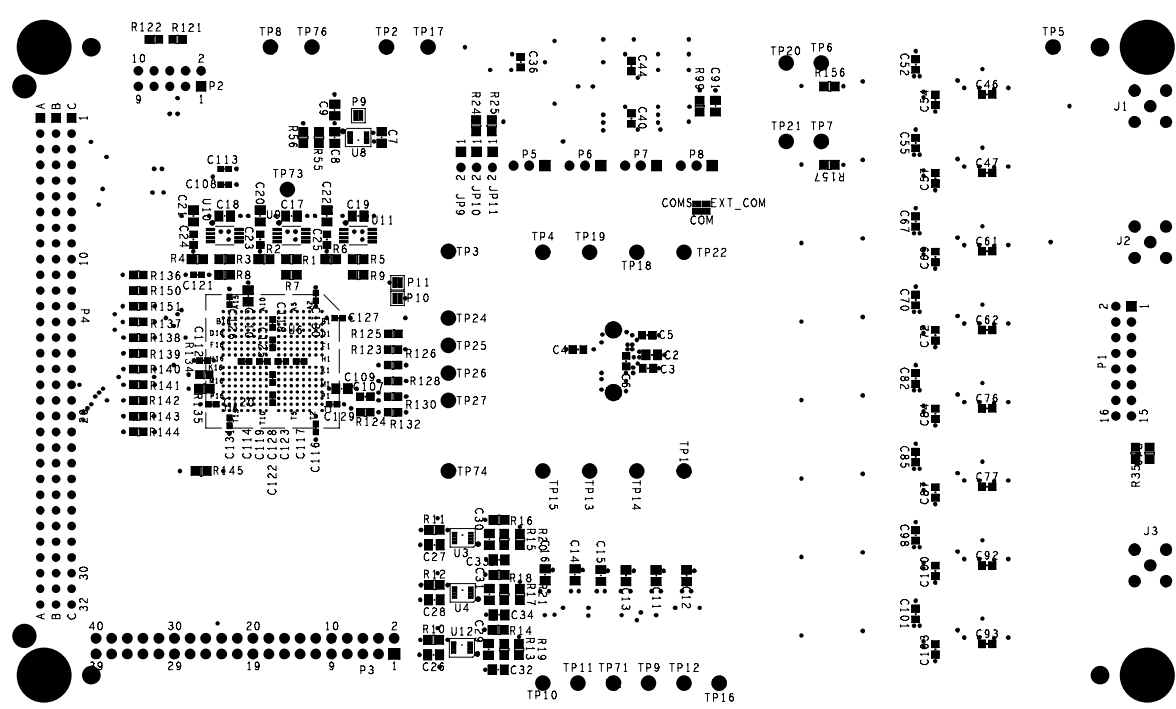
Figure 26. Bottom Layer
