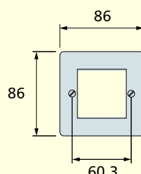
2 module K182 ALM
