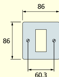
1 module K181 ALM
