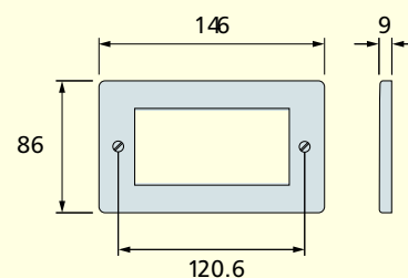
4 module K184 ALM
