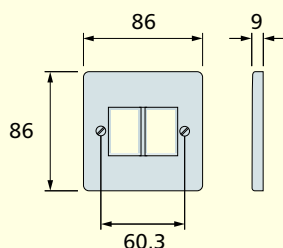
2 module K172 ALM
