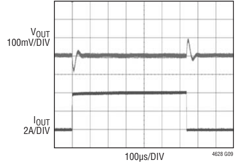
2.5V Load Transient
