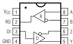
DIP/SO
