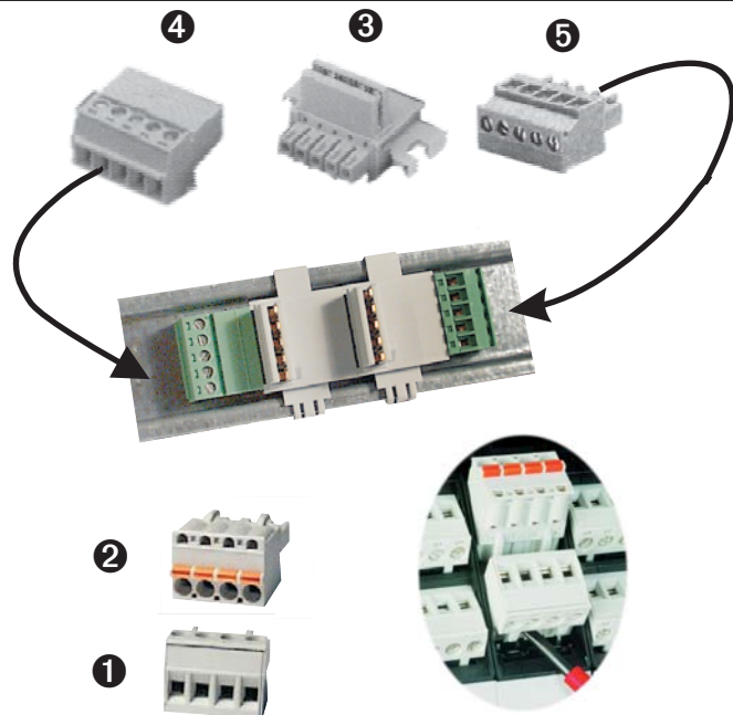
Bild 9: Zubehörteile
