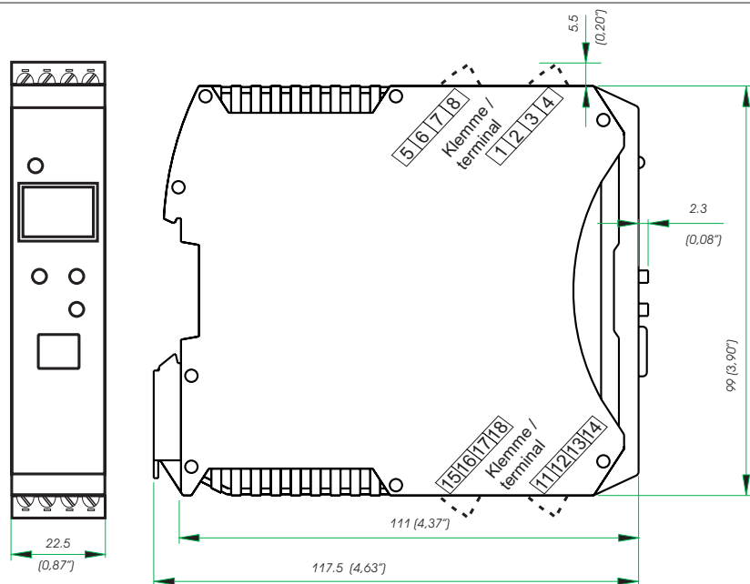
Bild 7: Abmessungen
