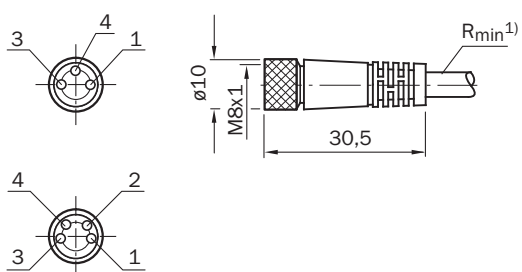
尺寸图 (尺寸单位: mm)
