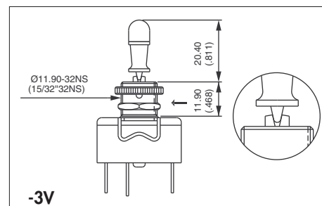
3 verriegelte Stellungen
