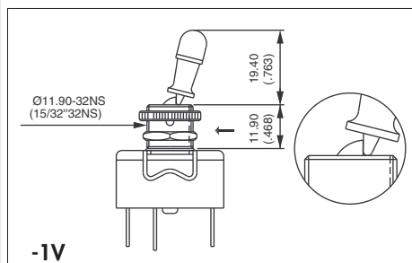
1 verriegelte Stellung
