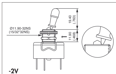
2 verriegelte Stellungen
