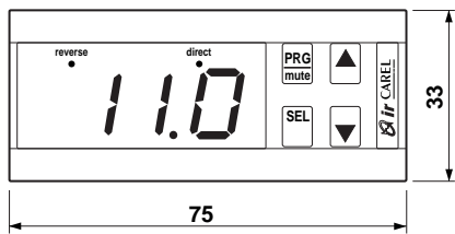
IR32 - montage encastré
