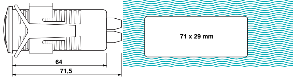
IR32 - Fronteinbau
